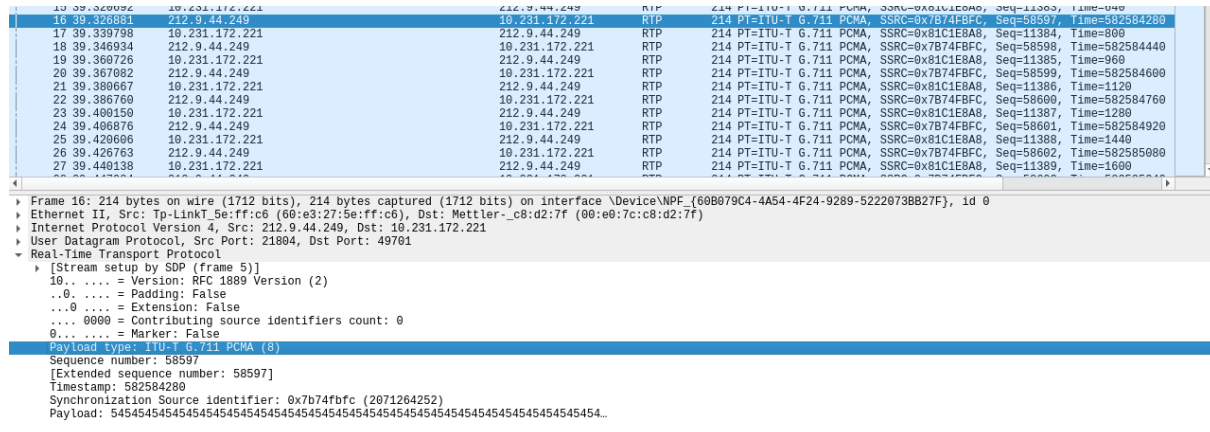
Abbildung 13: Auszug des RTP-Captures (Codec G.711)
