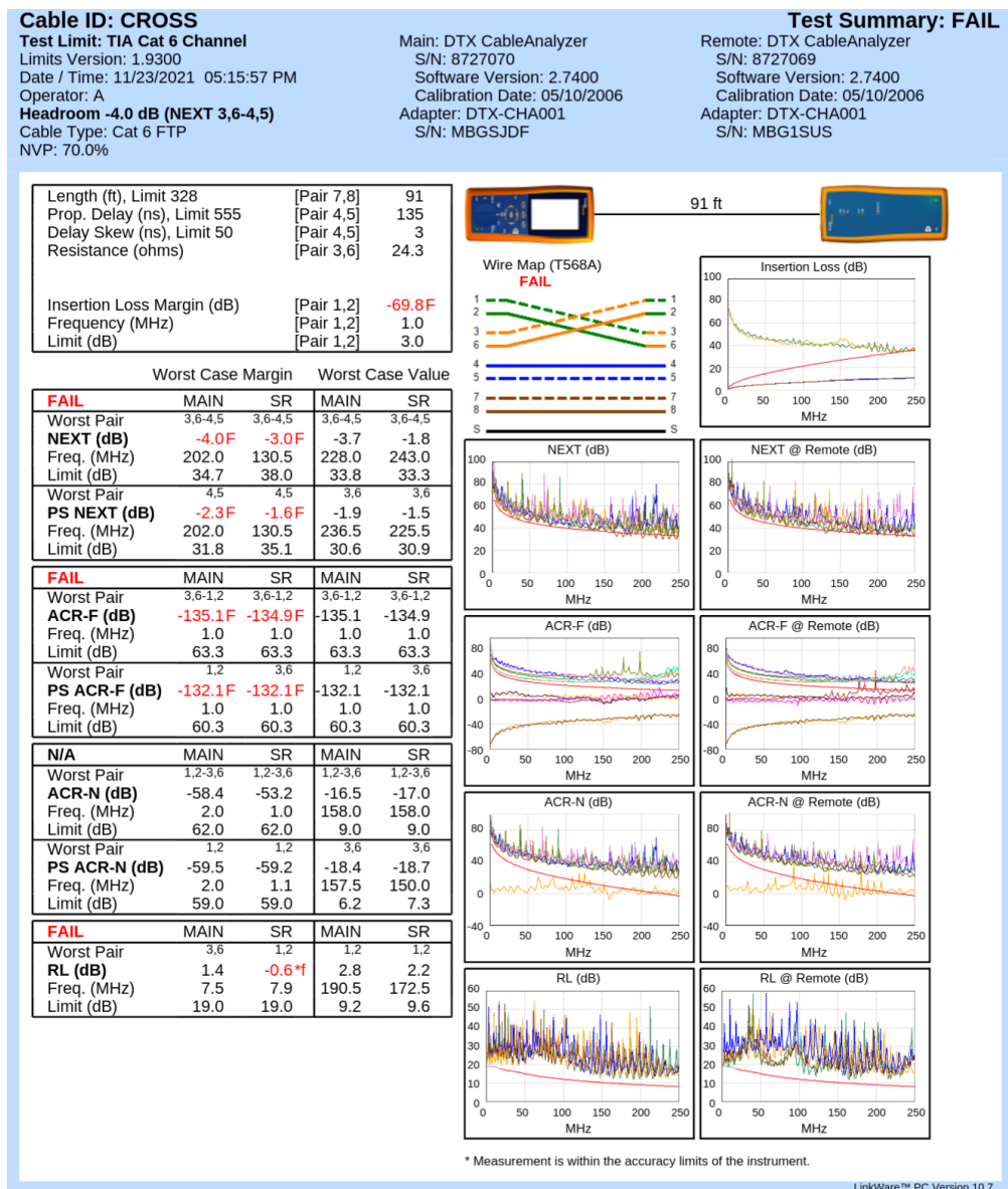
Abbildung 40: Ergebnisse der Messtechniker
