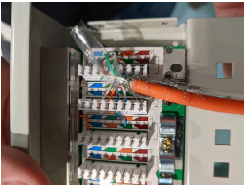
Abbildung 26: Patch-Panel-Verkabelung
