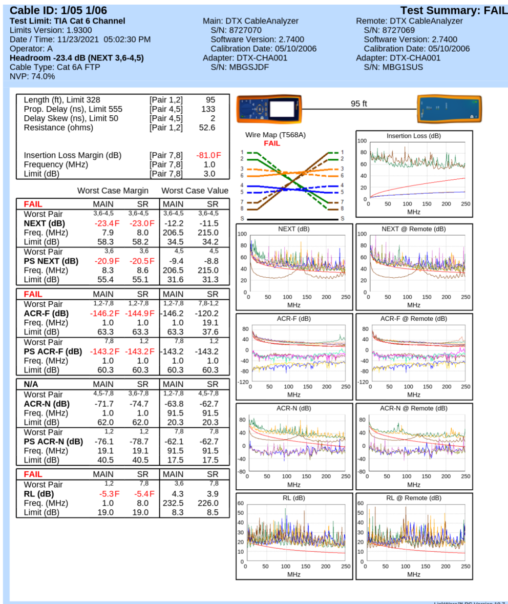
Abbildung 38: Ergebnisse der Messtechniker
