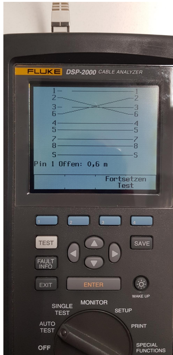
Abbildung 24: Ergebnis nach dem durchschneiden einer Ader
