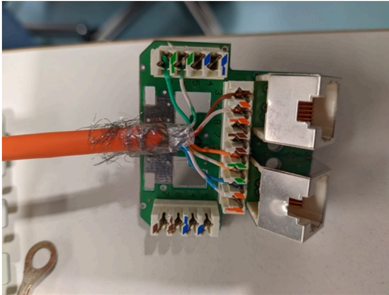
Abbildung 25: Buchsenverkabelung
