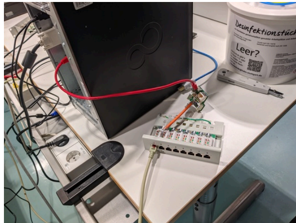
Abbildung 27: CableSharing mit der Workstation
