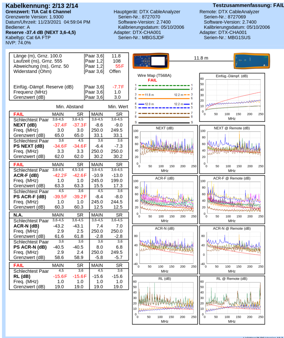
Abbildung 42: Ergebnisse der Messtechniker
