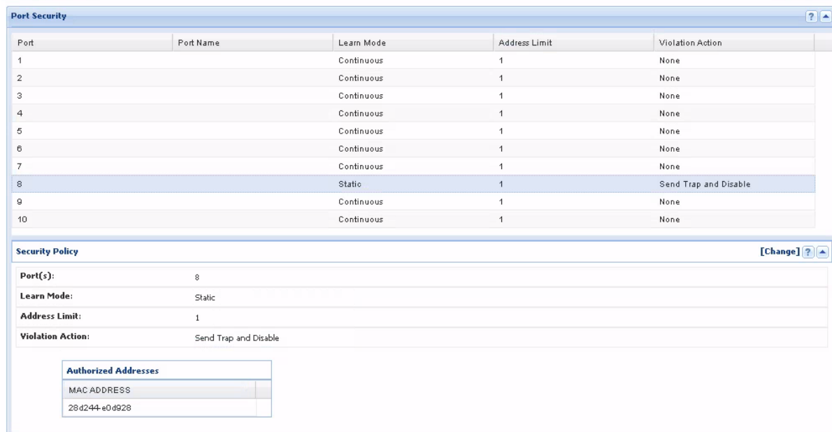
Abbildung 36: Aktivierte Port-Security auf Port 8 mit allowlistetem Laptop
