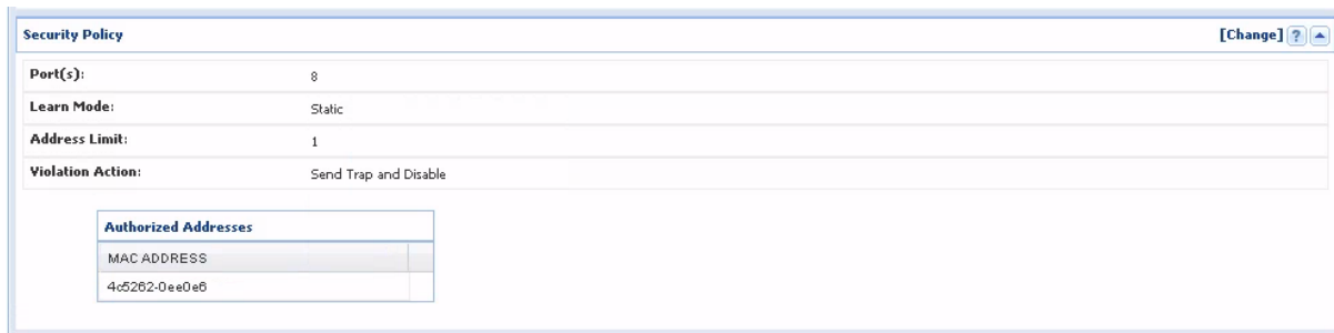
Abbildung 35: Aktivierte Port-Security auf Port 8 mit allowlisteter Workstation
